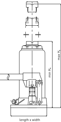
Jack dimensions
